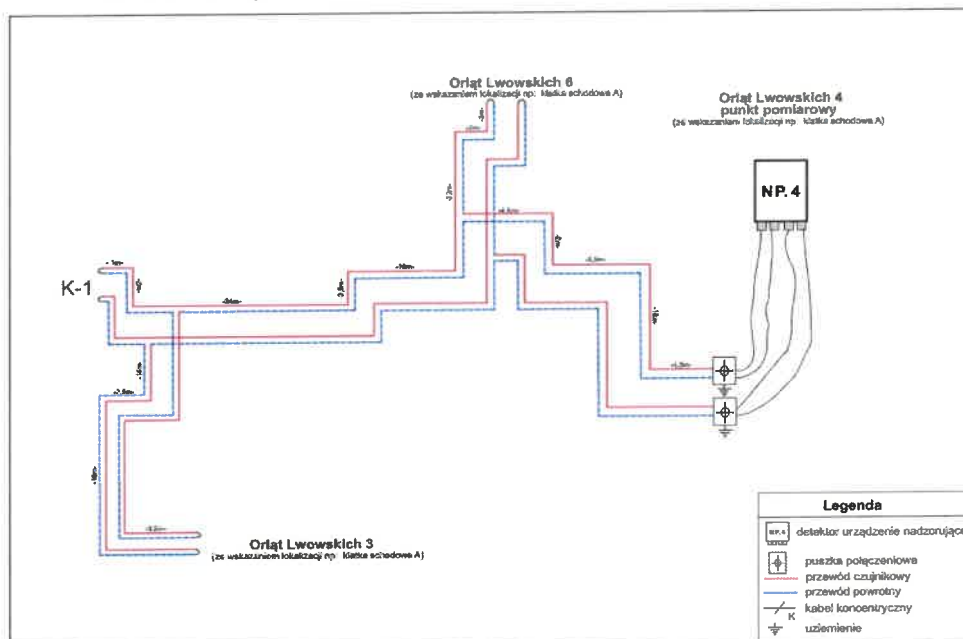
Rys. 2 Przykładowy schemat instalacji alarmowej
